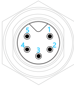
图 3 触发接口图
