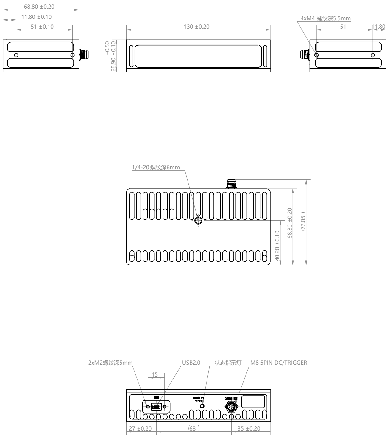
图 4 FM830-RI 尺寸图 (单位: mm)
