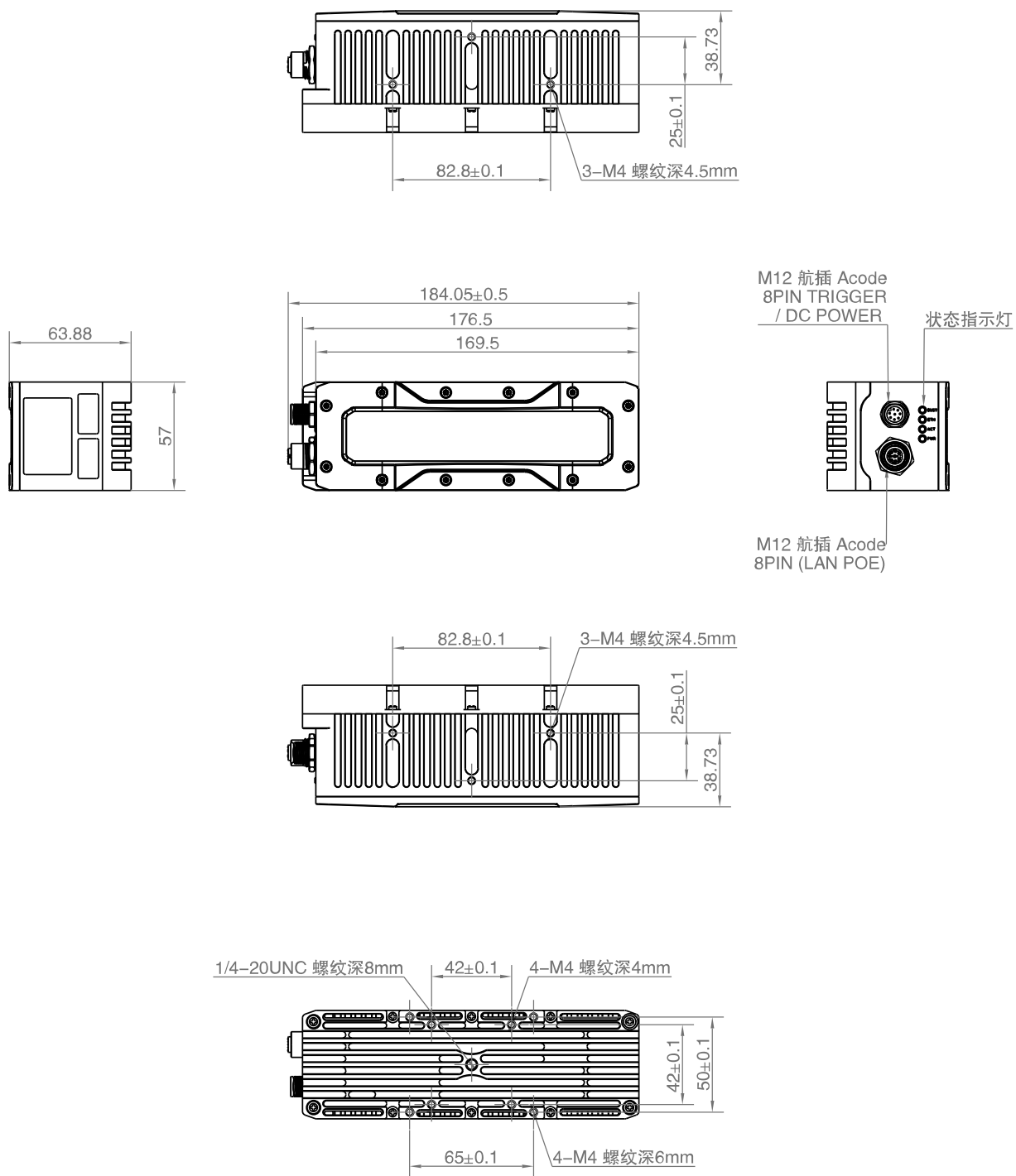
图 5 PS801 系列尺寸图 (单位: mm)
