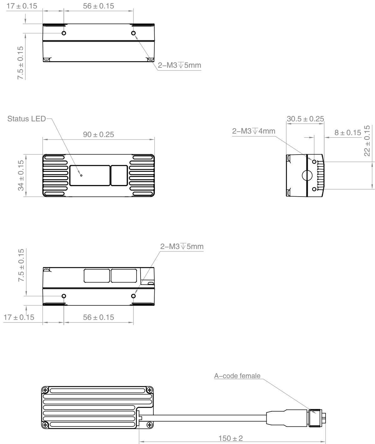
图4 TM260-E1 尺寸图 (单位: mm)
