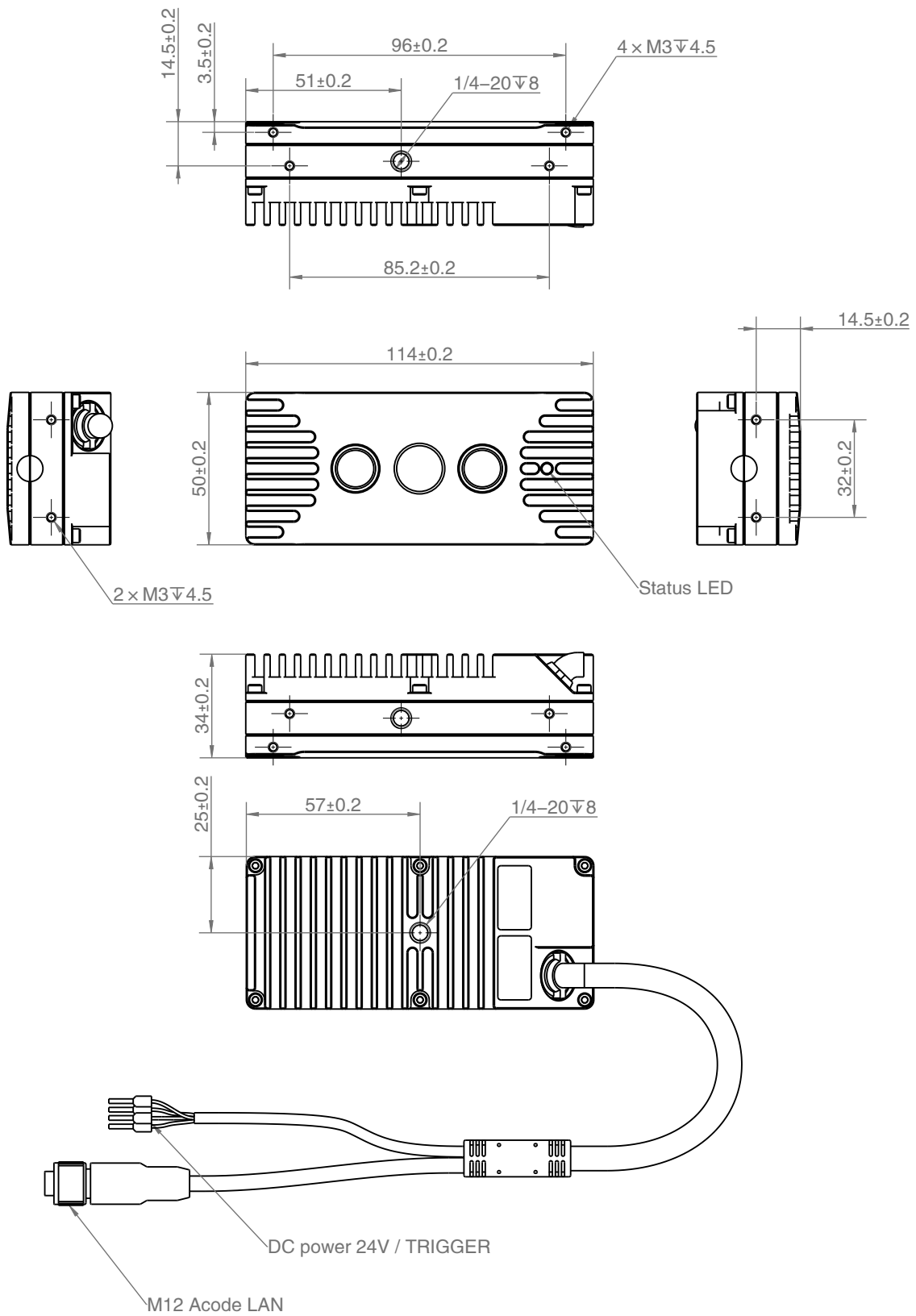
图 3 TM421-E1 尺寸图 (单位: mm)
