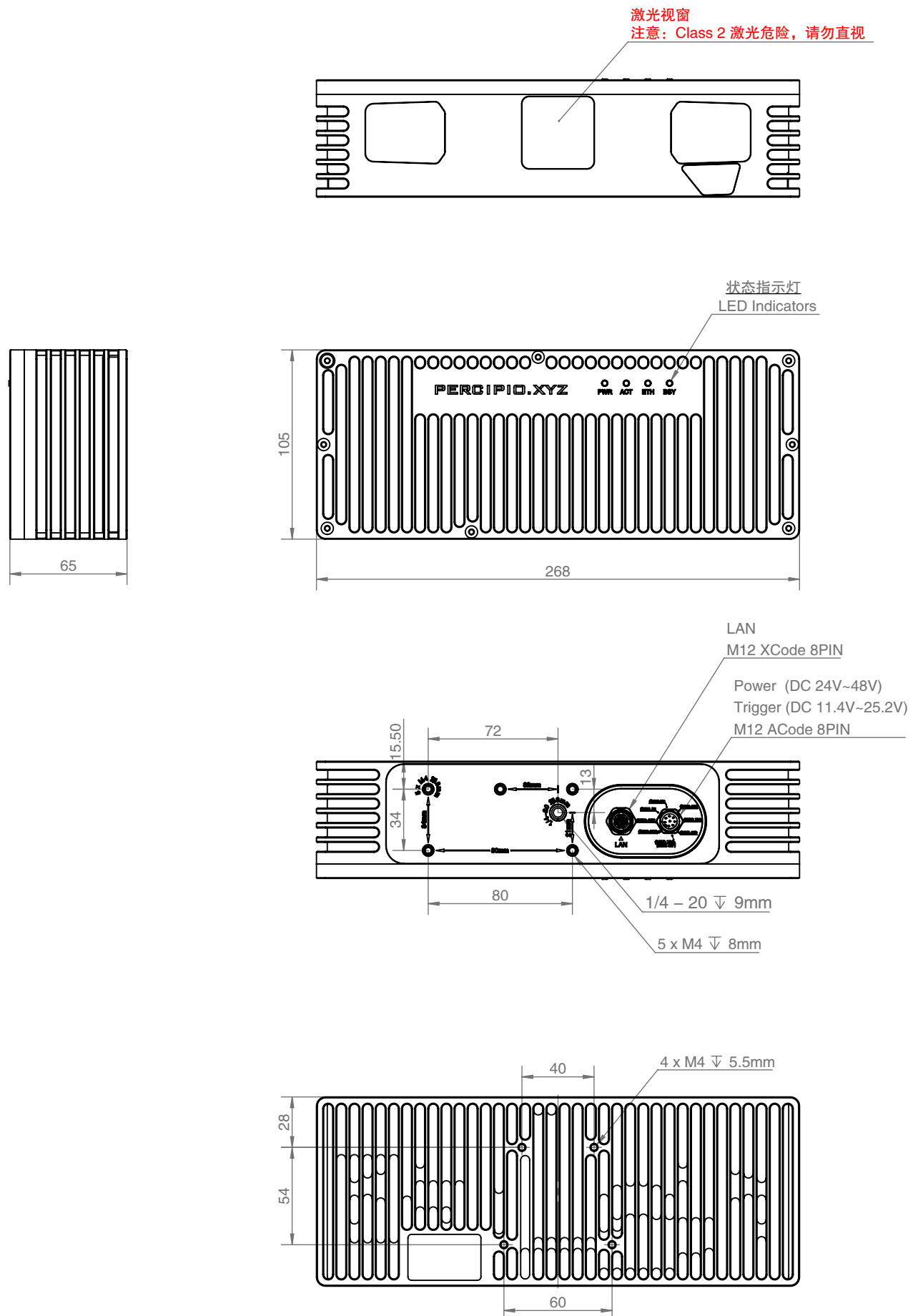
图 4 VMD02-4070 尺寸图 (单位: mm)
