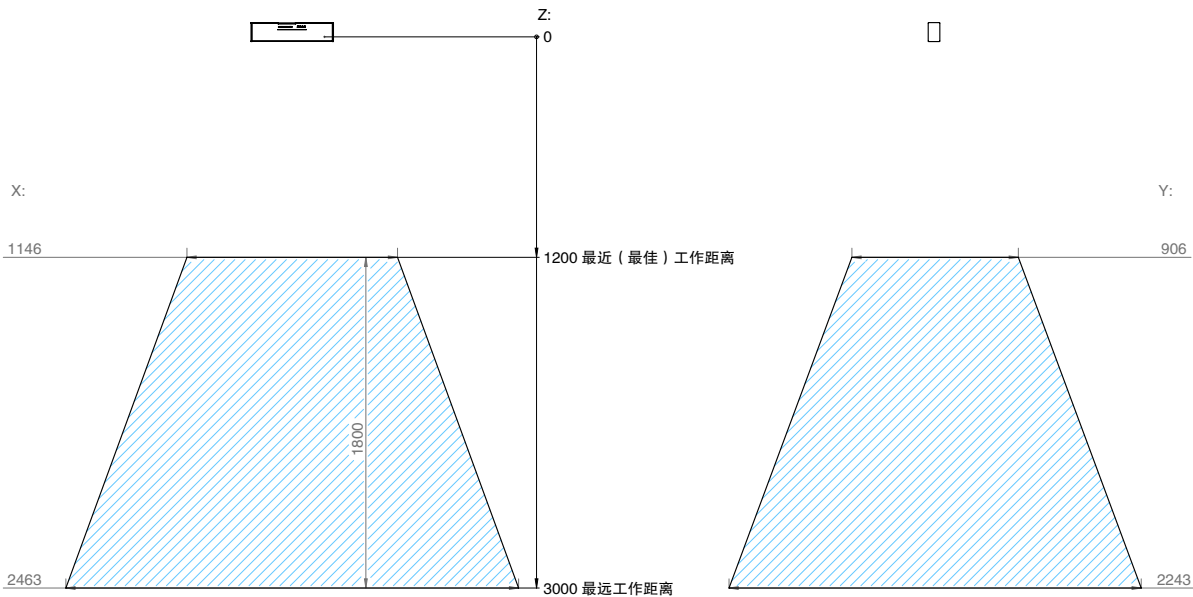
图 1 FOV (单位：mm)
