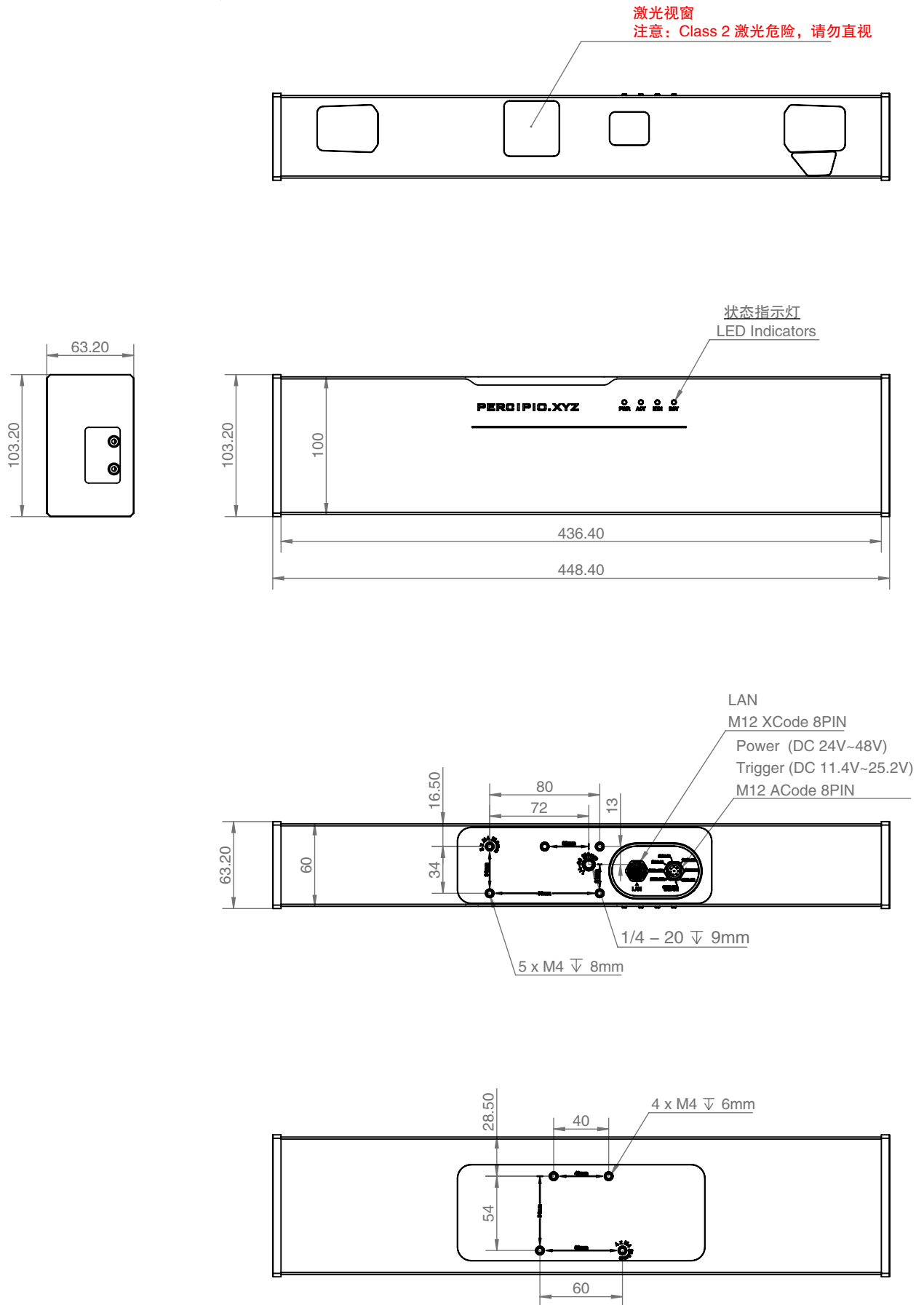
图 4 VMD03-1230C \ VMD03-1230 尺寸图 (单位: mm)
