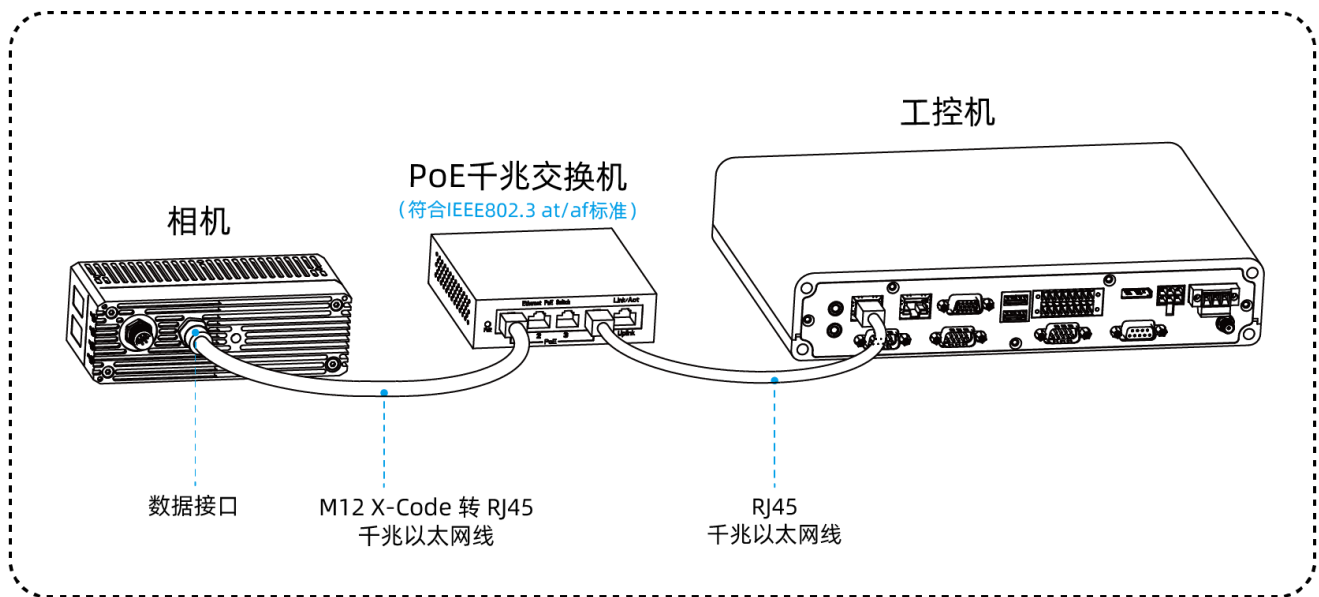
图 6 连接方式 2
