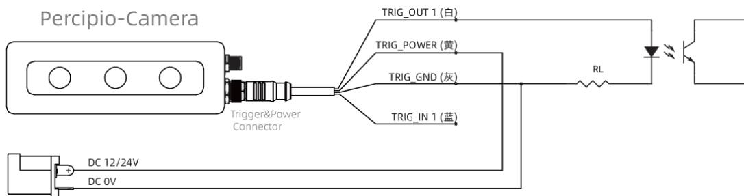
图 9 上升沿触发输出接线参考—驱动光耦
